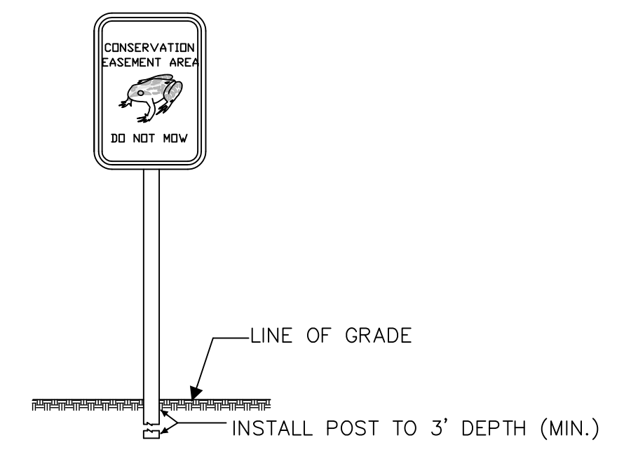
NO-MOW AREA SIGN DETAIL N.T.S.
